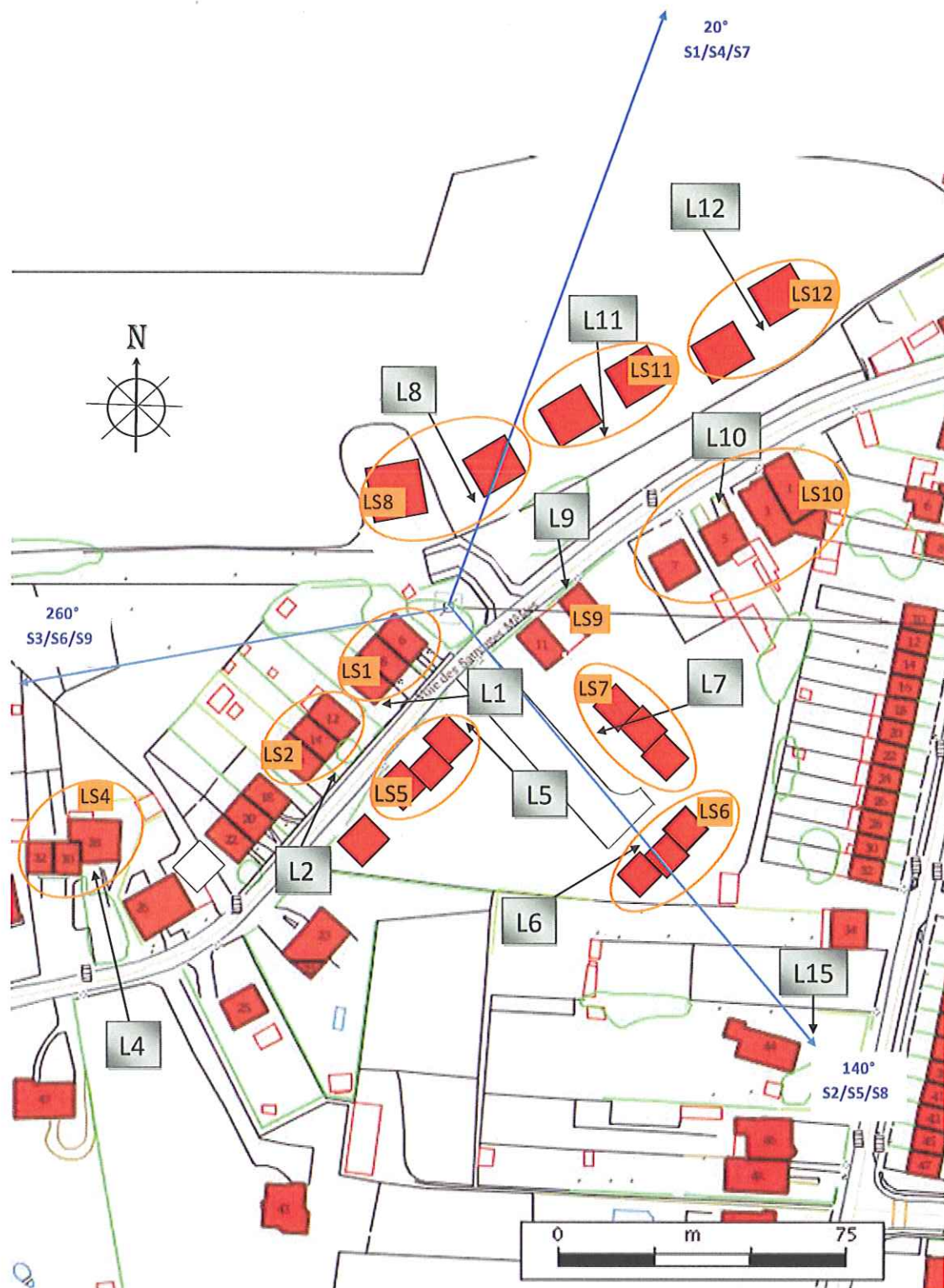
Figure 1 : Plan de la zone autour de l'antenne.
