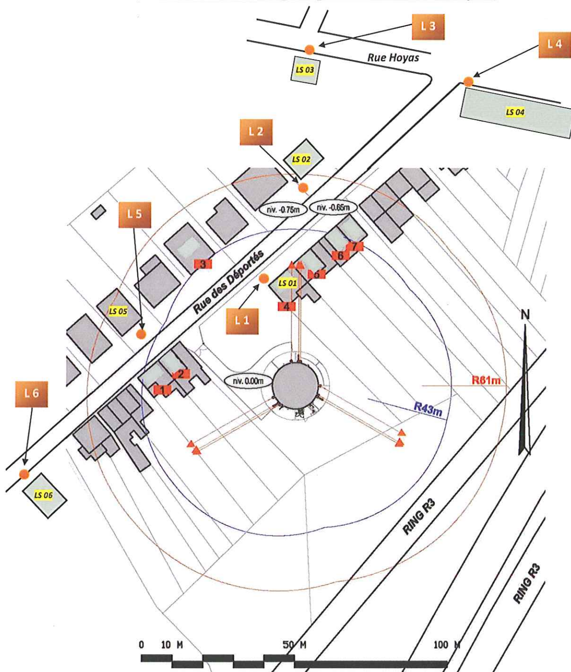
Figure 1 : Plan de la zone autour de l'antenne.
