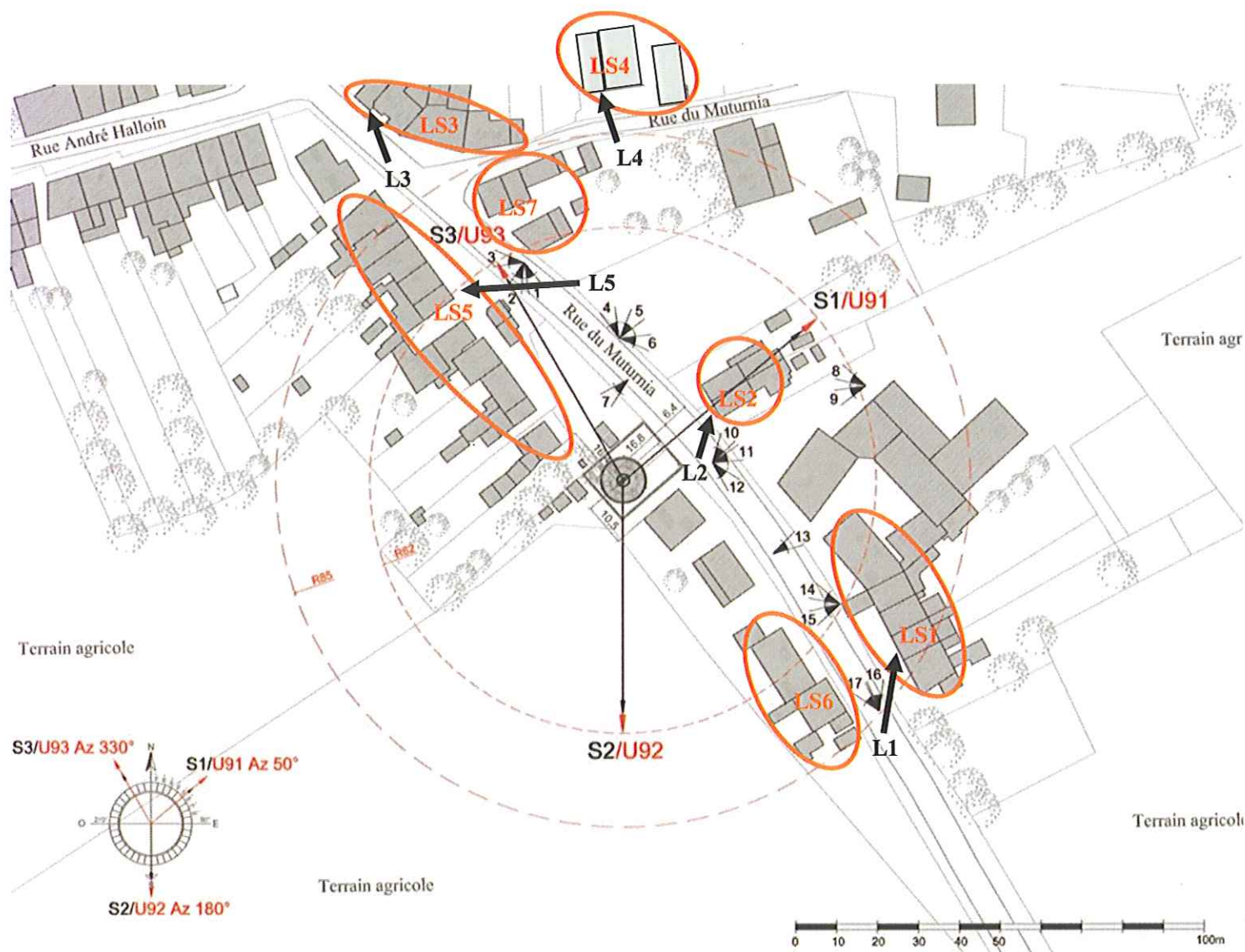
Figure 1 : Plan de la zone autour de l'antenne.
