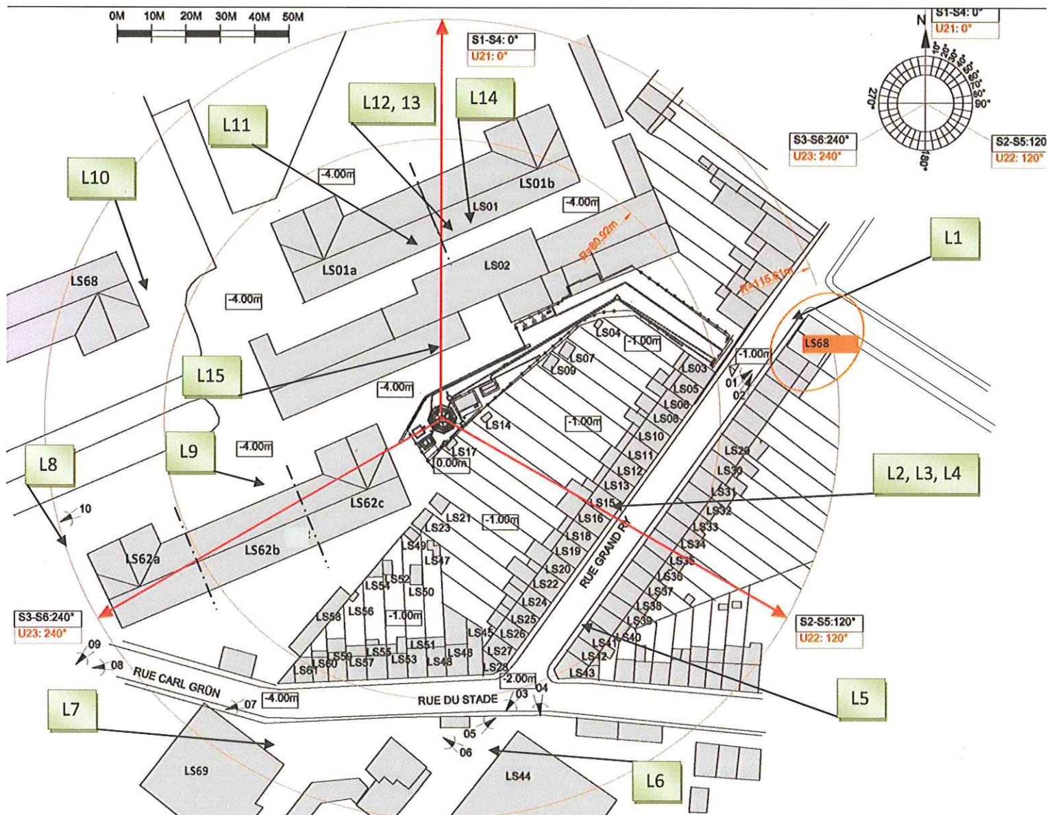
Figure 1 : Plan de la zone autour de l'antenne.
