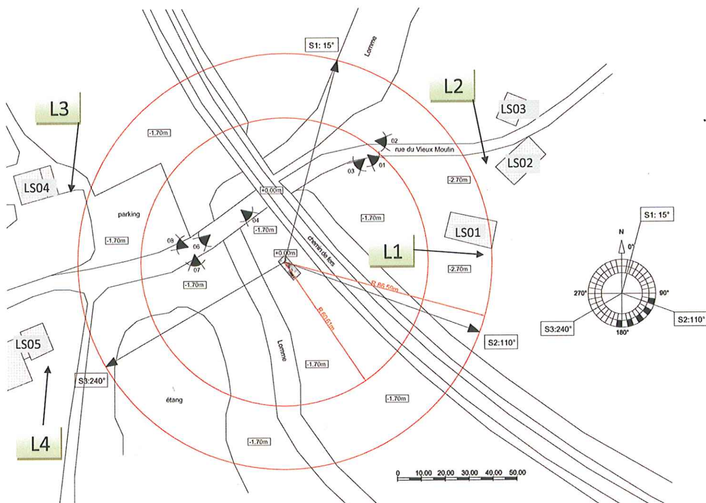
Figure 1 : Plan de la zone autour de l'antenne.
