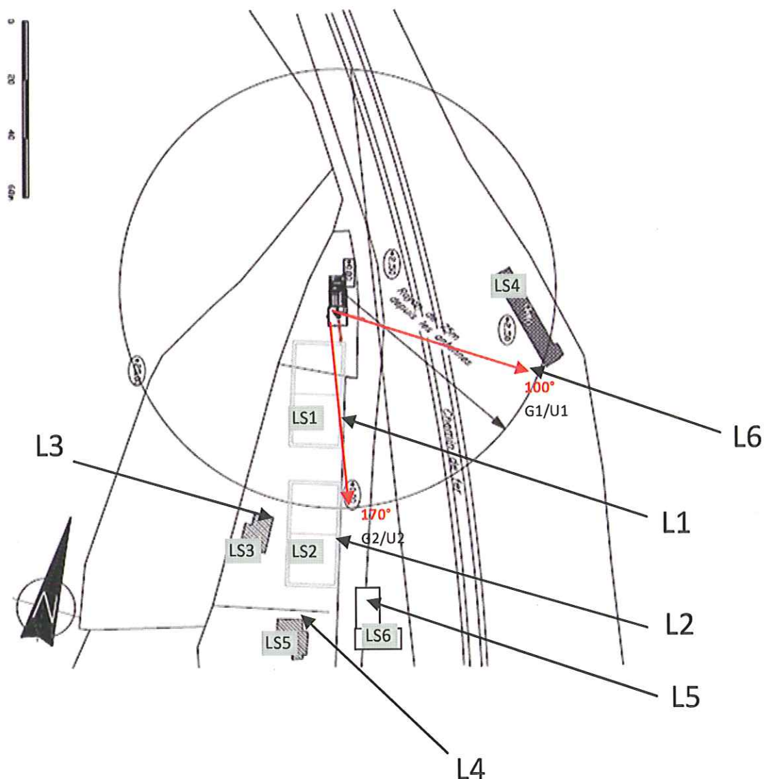
Figure 1 : Plan de la zone autour de l'antenne.
