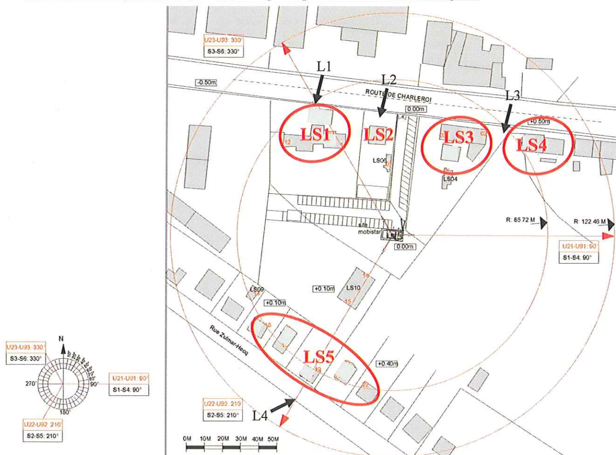
Figure 1 : Plan de la zone autour de l'antenne.
