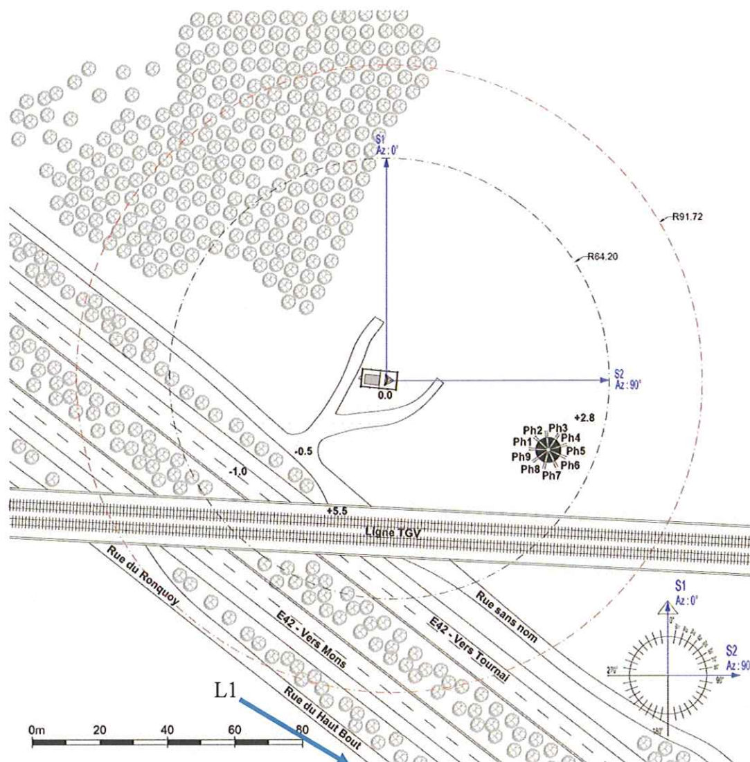
Figure 1 : Plan de la zone autour de l'antenne.
