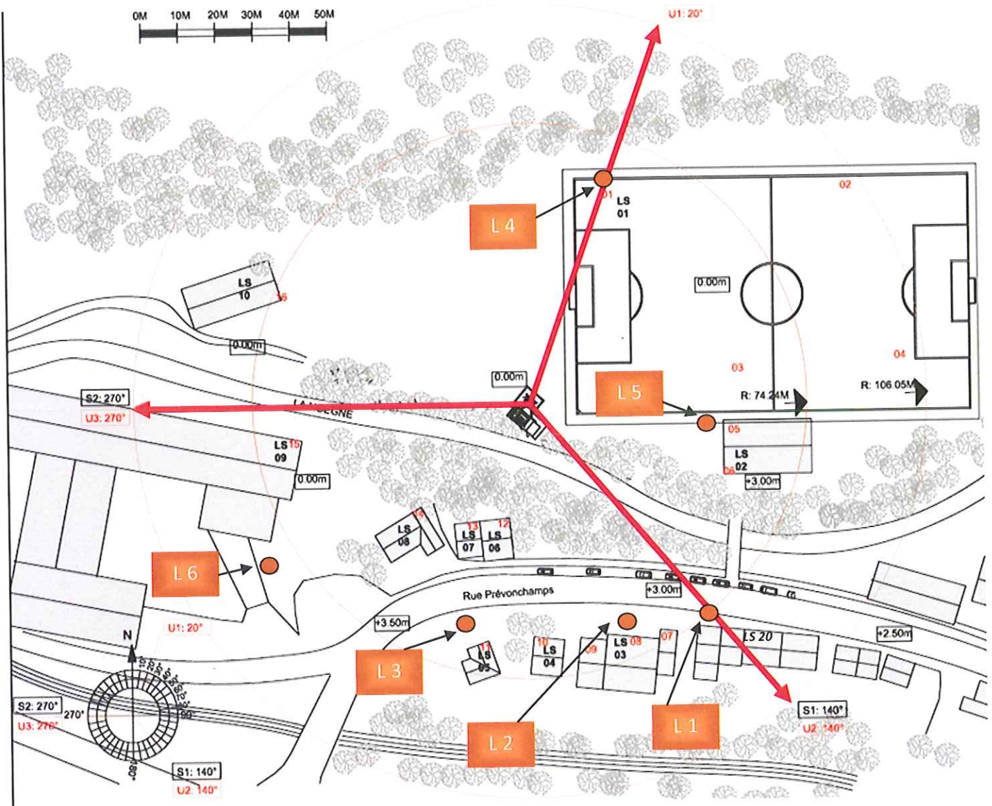
Figure 1 : Plan de la zone autour de l'antenne.
