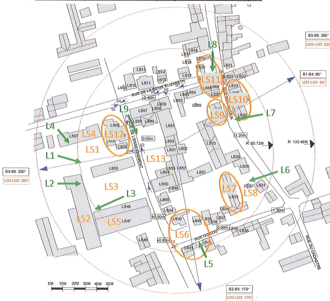
Figure 1 : Plan de la zone autour de l'antenne.
