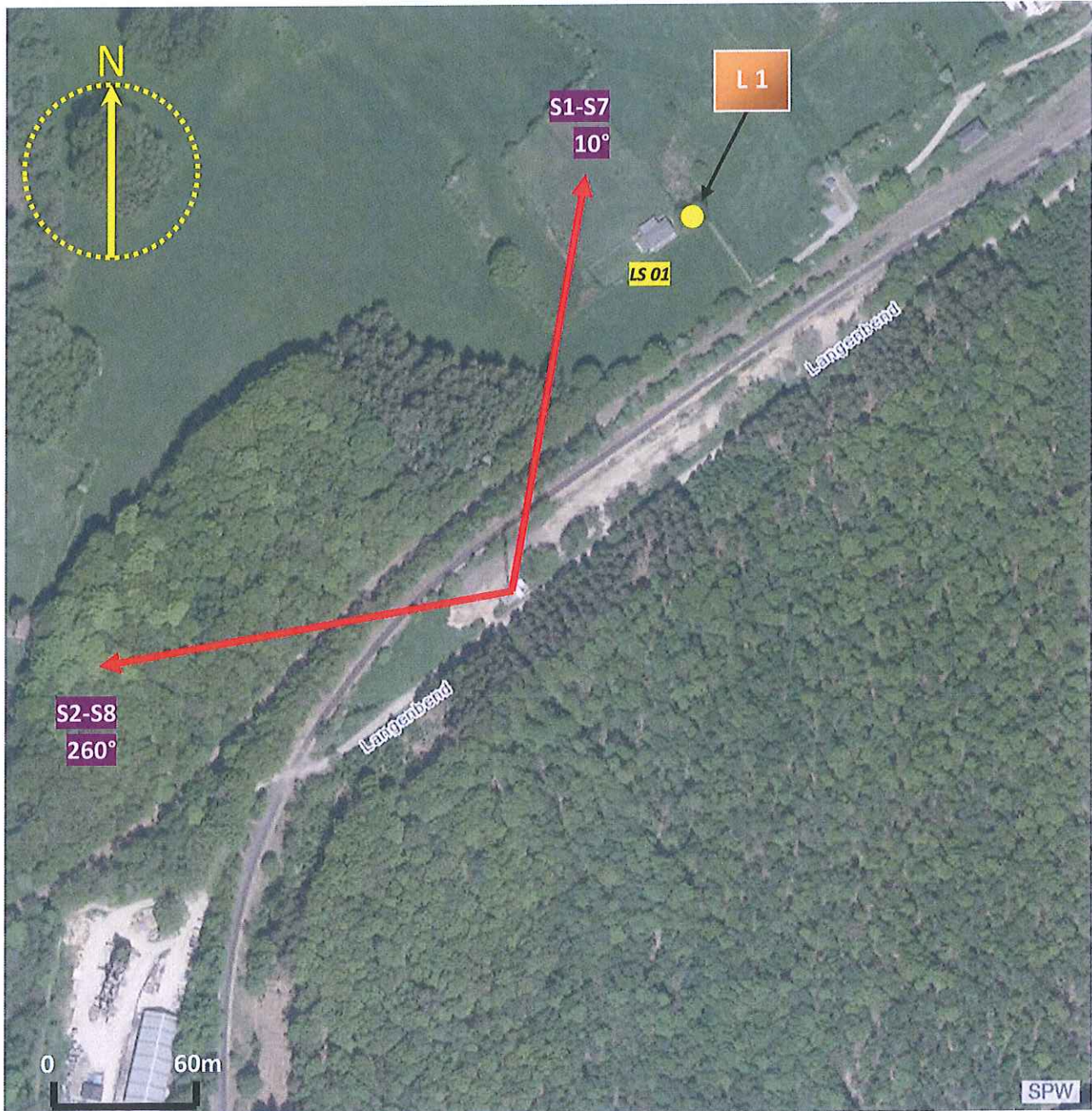
Abbildung 1 : Plan der Zone im Umkreis der Antenne
