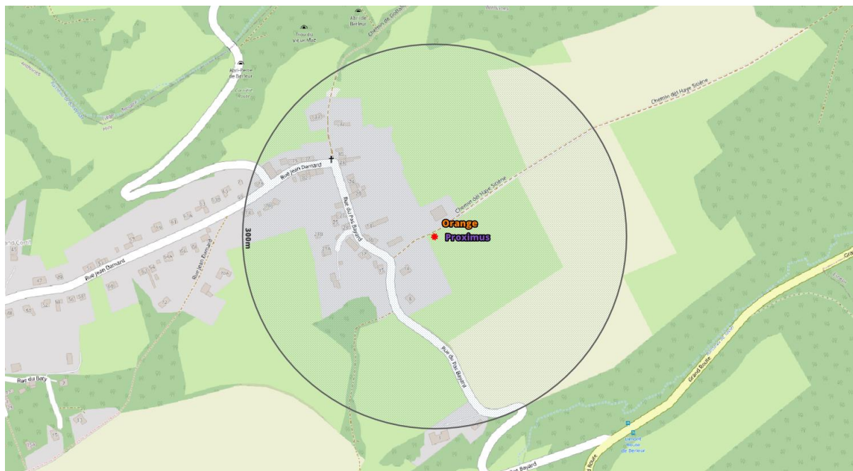
Figure 2 : Vue en plan des installations d'antennes dans un rayon de 300 mètres autour de l'installation faisant l'objet de la demande d'avis
