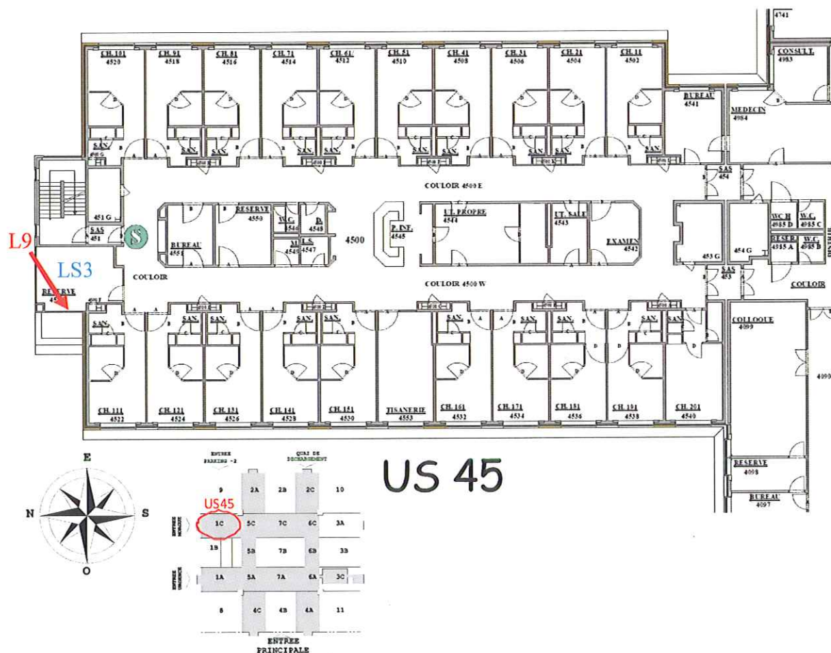
Figure 3 : 4 ème étage – Coté nord-est – US 45
