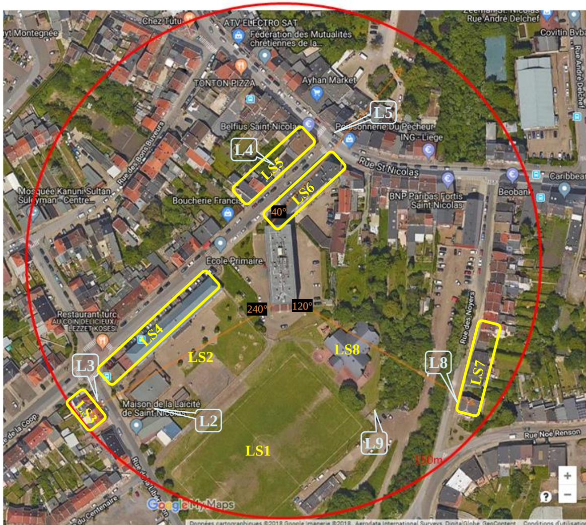
Figure 1 : Plan de la zone autour de l'antenne.
