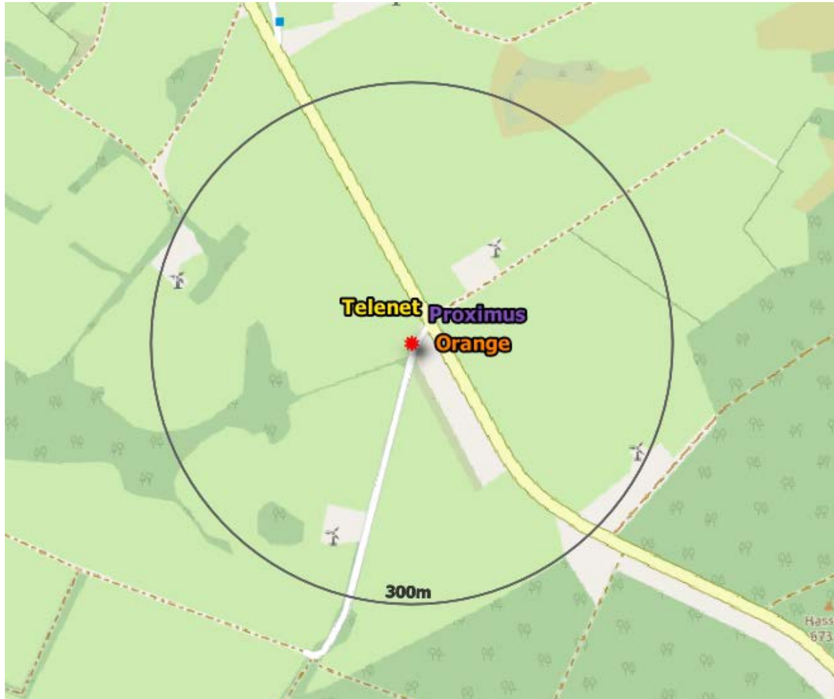
Abbildung 3: Planansicht der Antennenanlagen in einem Radius von 300 Metern um die Anlage, die Gegenstand des Antrags auf Stellungnahme ist
