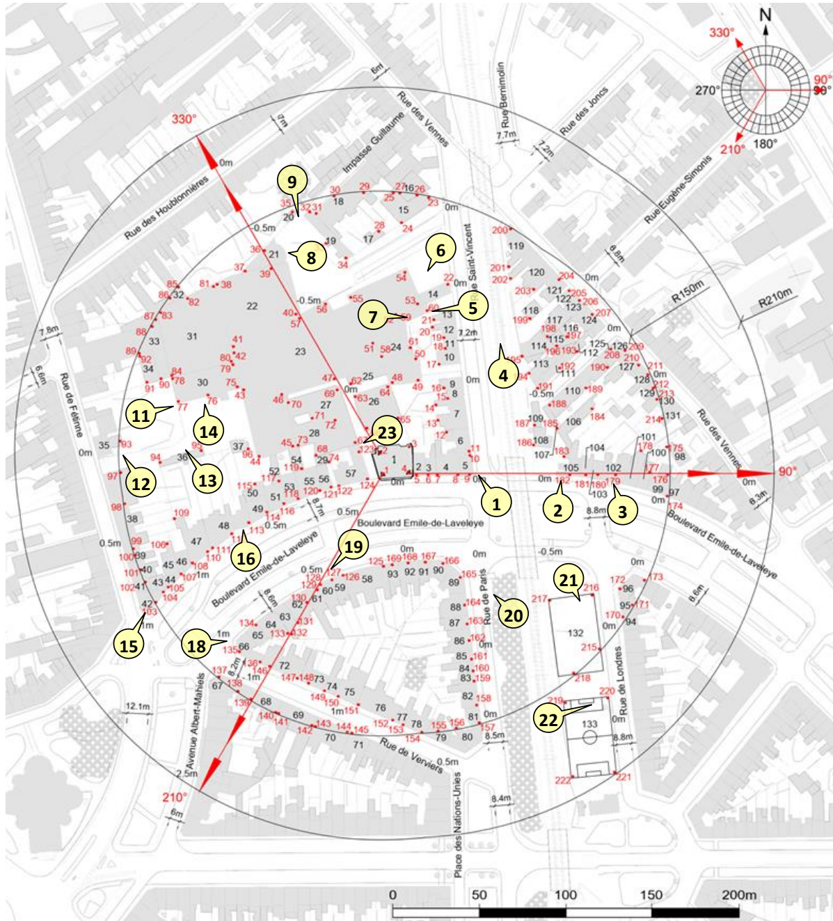
Figure 1 : Plan de la zone autour de l'installation.
