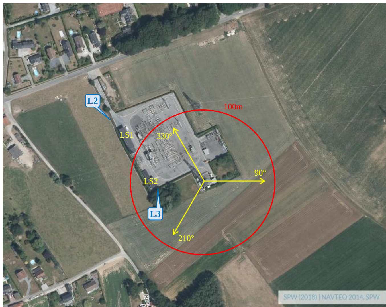
Figure 1 : Plan de la zone autour de l'antenne.
