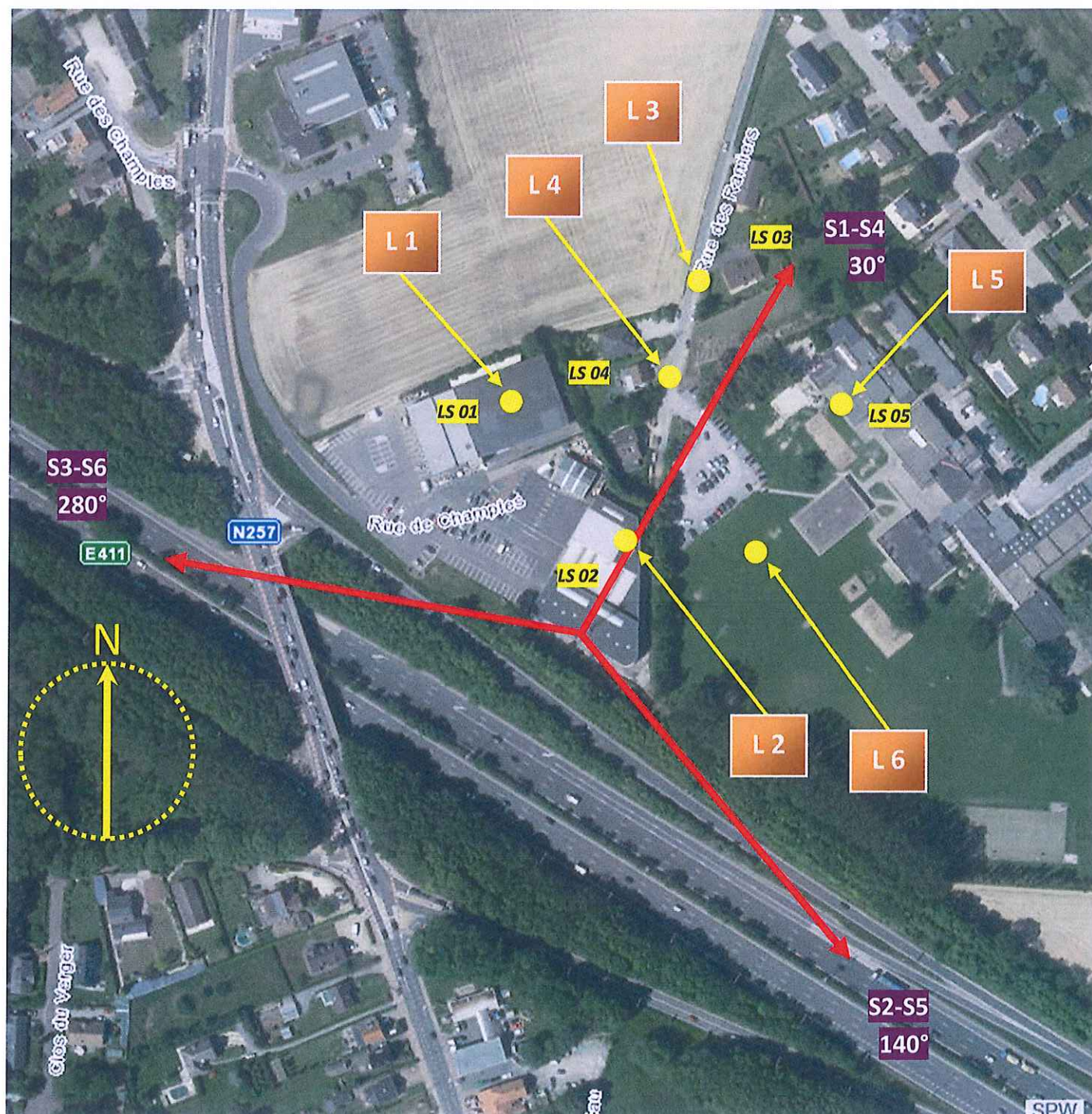
Figure 1 : Plan de la zone autour de l'antenne.
