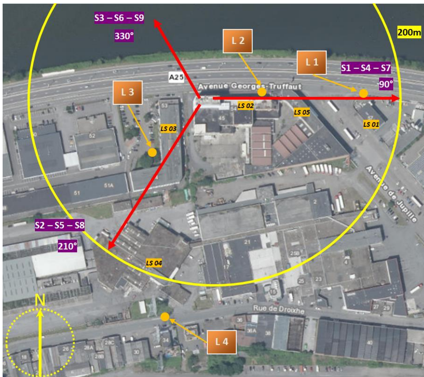
Figure 1 : Plan de la zone autour de l'antenne.
