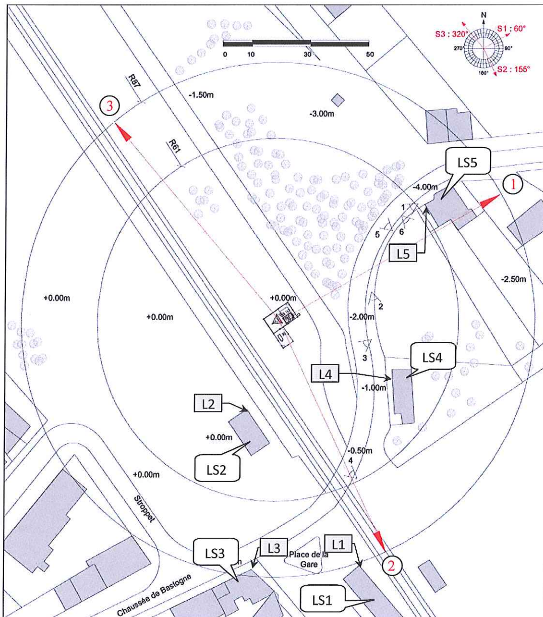
Figure 1 : Plan de la zone autour de l'antenne.
