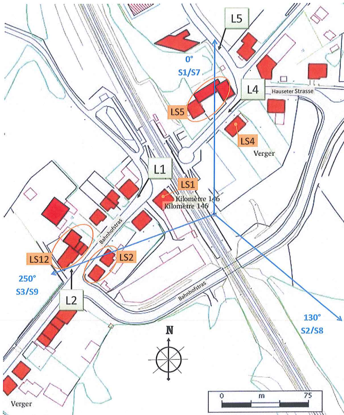
Abbildung 1 : Plan der Zone im Umkreis der Antenne
