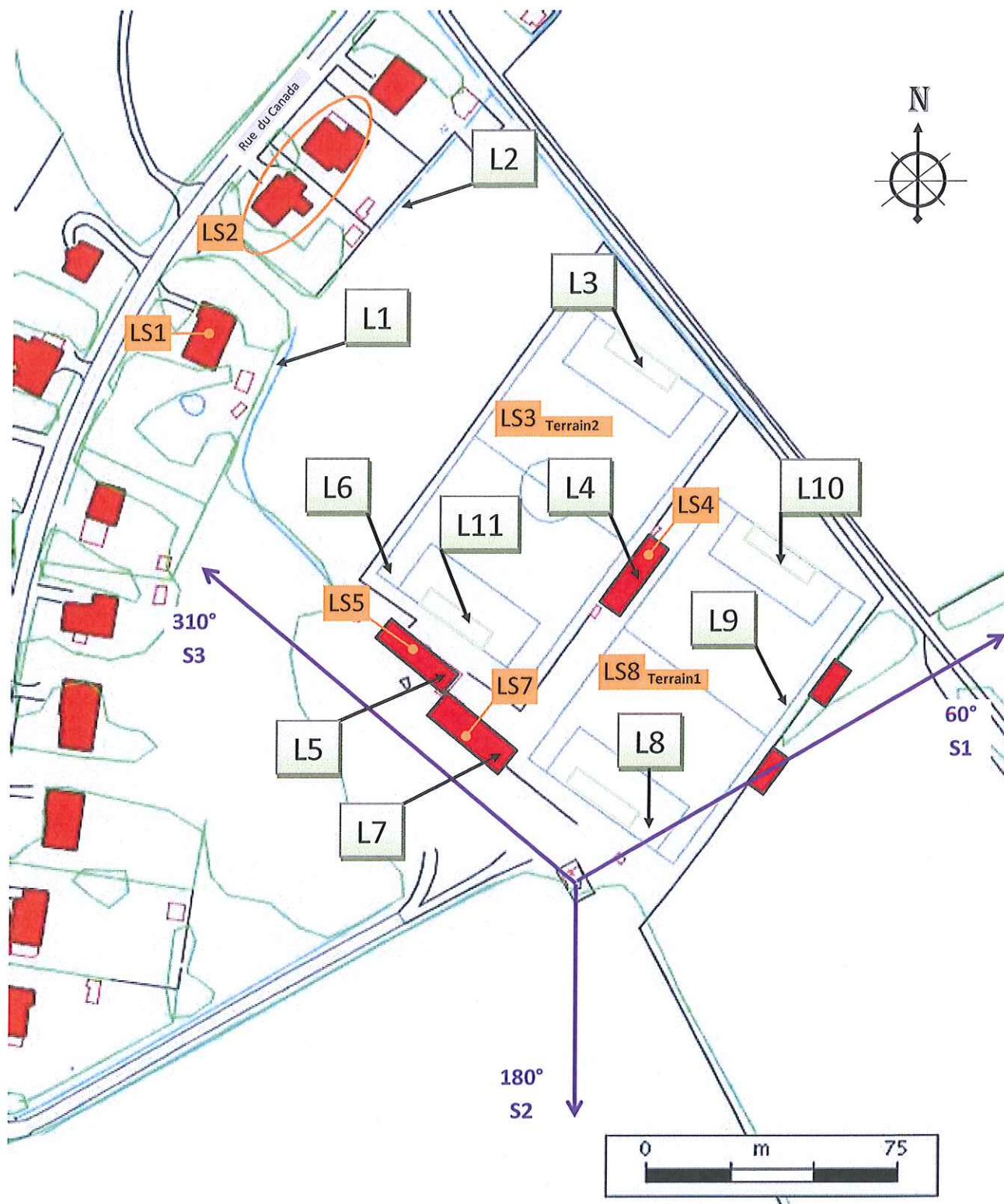
Figure 1 : Plan de la zone autour de l'antenne.
