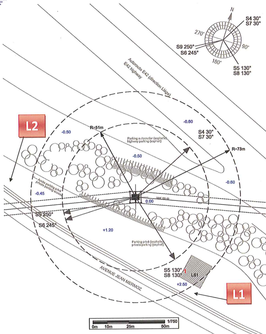
Figure 1 : Plan de la zone autour de l'antenne.
