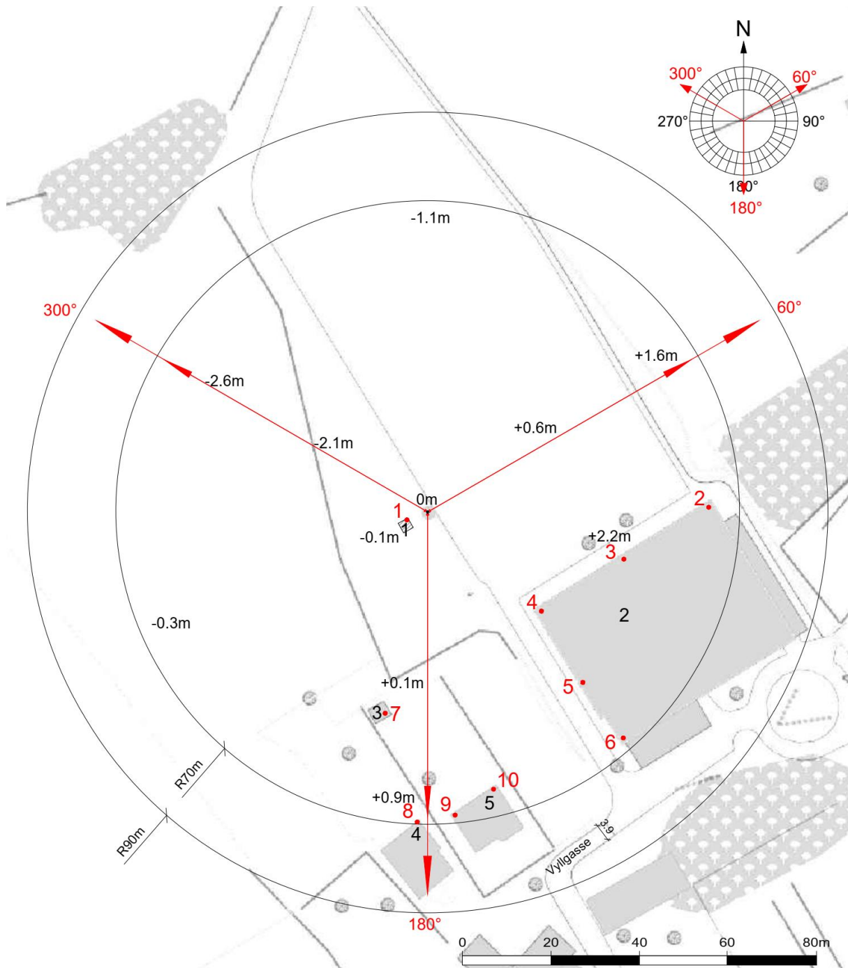
Abbildung 1: Draufsicht der Aufenthaltsräume und der Kontrollpunkte
