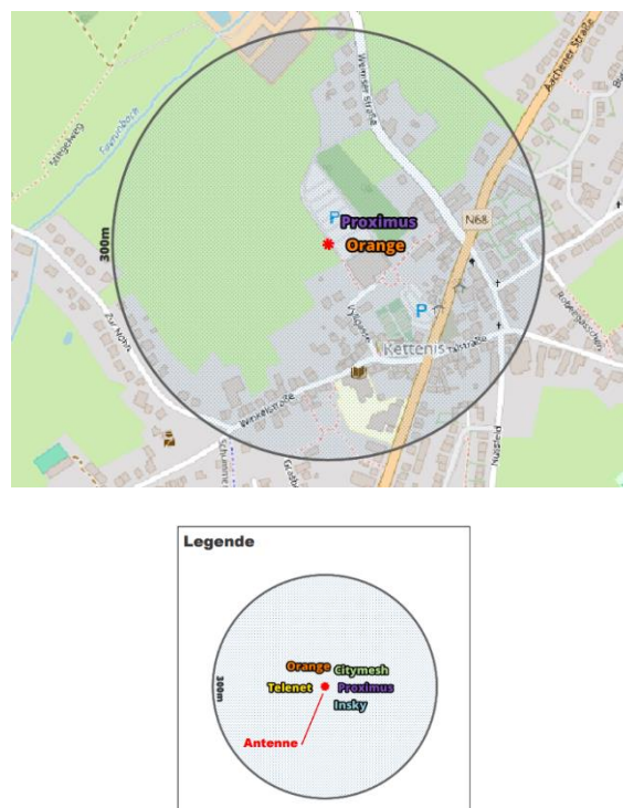
Abbildung 3: Planansicht der Antennenanlagen in einem Radius von 300 Metern um die Anlage, die Gegenstand des Antrags auf Stellungnahme ist
