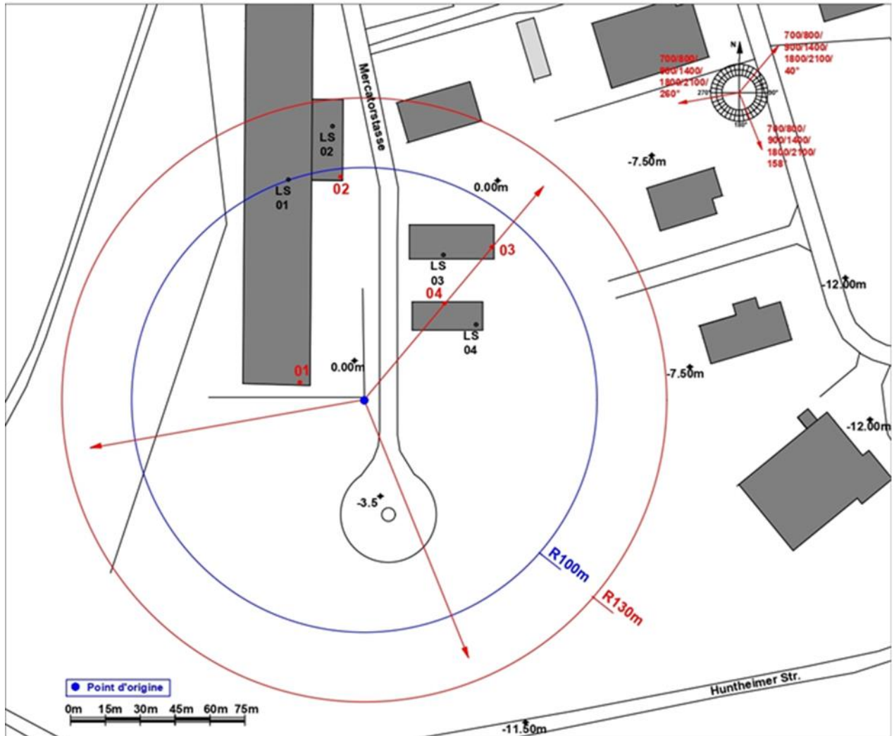
Abbildung 1: Draufsicht der Aufenthaltsräume und der Kontrollpunkte
