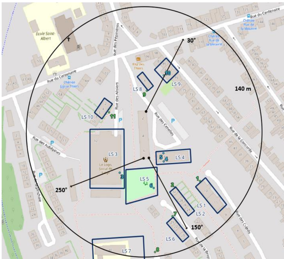
Figure 1 : Plan de la zone autour de l'installation.
