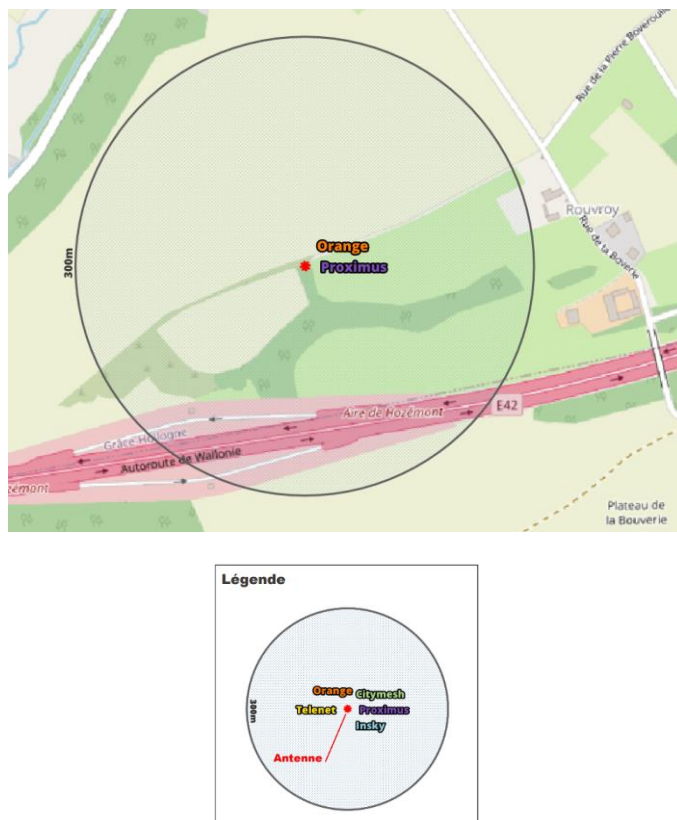
Figure 2 : Vue en plan des installations d'antennes dans un rayon de 300 mètres autour de l'installation faisant l'objet de la demande d'avis
